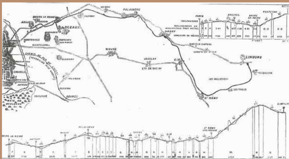
Plan et profil en long de la ligne à son extension maximale en voie large
