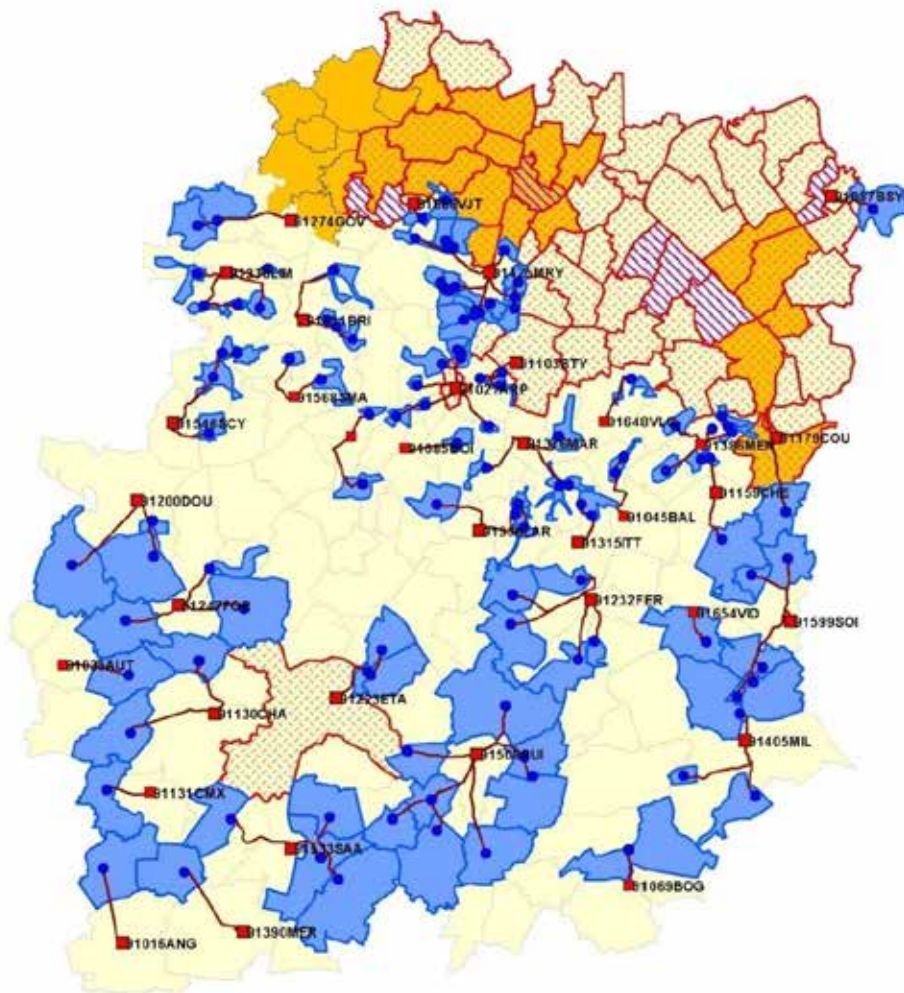
CG91 - Montée en Débit (MeD) Source France Télécom - Traitement Loopgrade ■ Contour des SR éligibles à la MeD (116) ■ Position des SR éligibles à la MeD ■ Position des NRA éligibles à la MeD — Segments NRA-SR ▨ Communes ZTD ARCEP ▨ Communes concernées par une intention de déploiement FTTH privé ■ Communes concernées par un RIP
